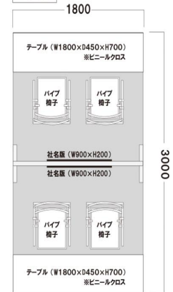
平面図
